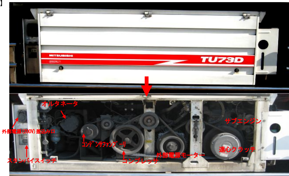
写真 4. 79 三菱重工製パワーユニット（セパレート型）
