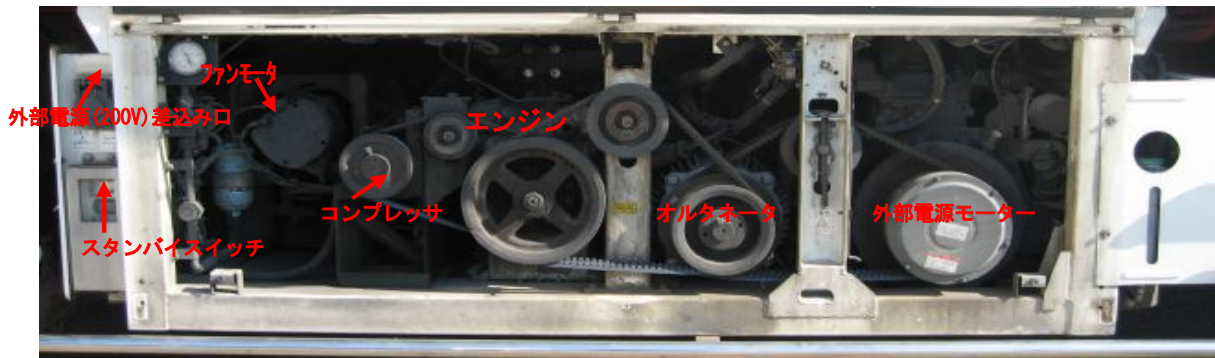
写真 4. 79 三菱重工製パワーユニット（セパレート型）
